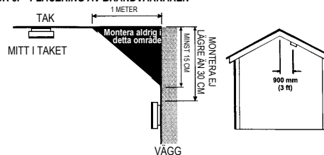
FIGUR 3i – PLACERING AV BRANDVARNAREN
